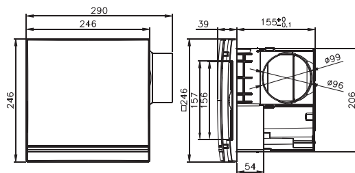
外觀尺寸圖 (mm)
